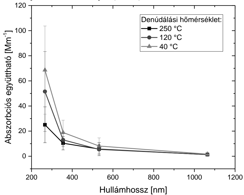
1. ábra Az abszorpciós együttható változása a denudálási hőmérséklet függvényében
